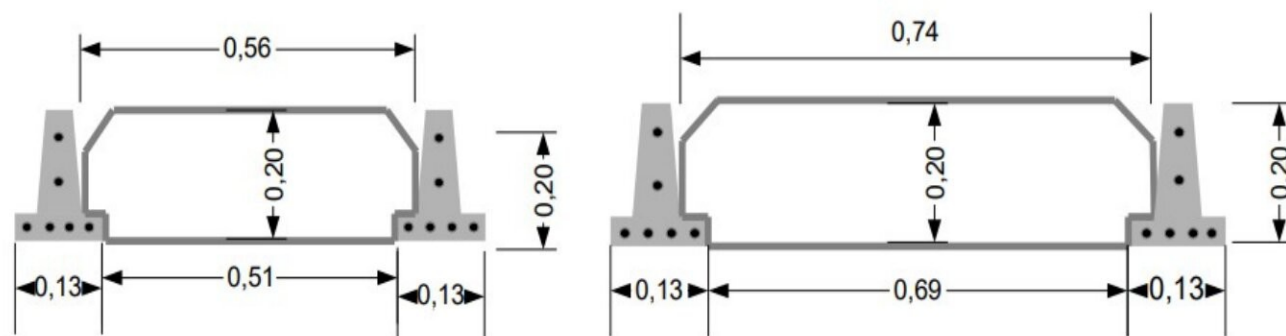
Diagrama de Vigueta pretensada 20-6
